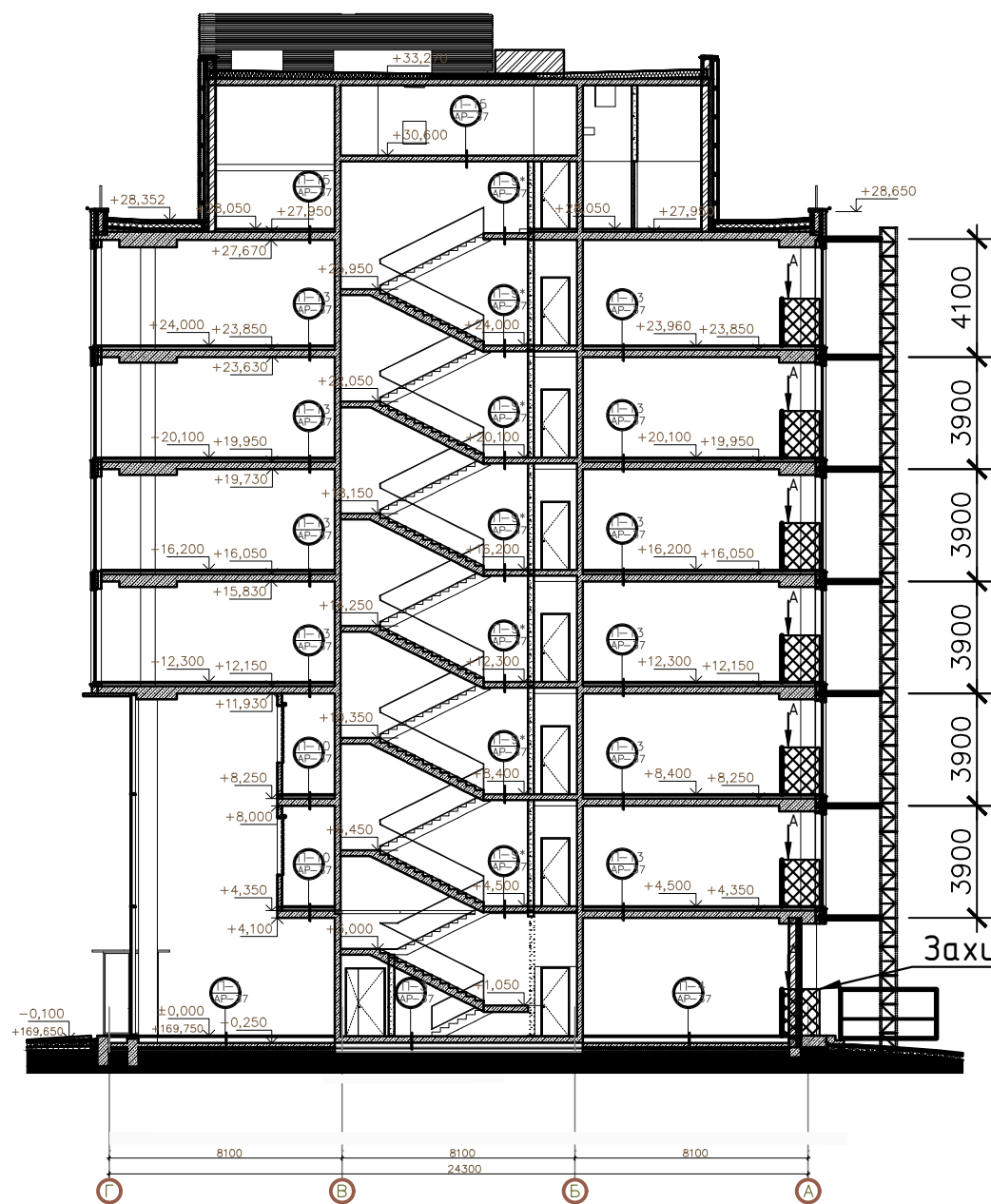
Вид А
