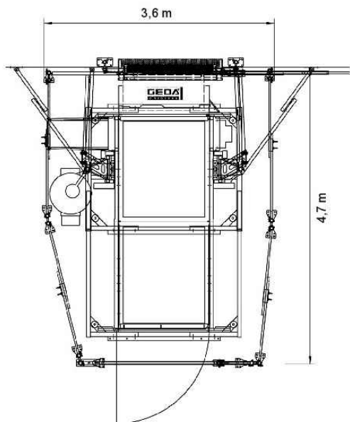
Platzbedarf am Beispiel Bühne „B“ mit Umwehrung / Example for space requirement platform „B“ with base enclosure
