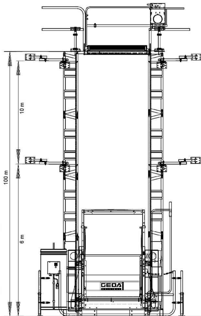
Platzbedarf am Beispiel Bühne „B“ mit Umwehrung / Example for space requirement platform „B“ with base enclosure
