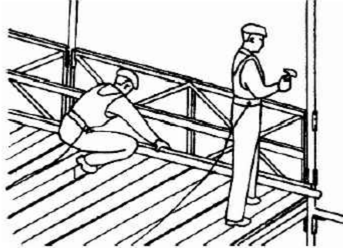
Установка елементів огорожі на третьому ярусі
