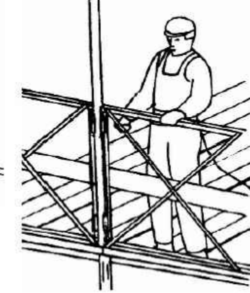
Зняття елементів огорожі на другому ярусі
