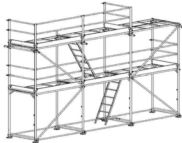
Влаштування сходів для переміщення працівників між ярусами
