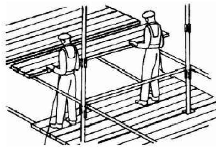
Зняття щитів настилу на другому ярусі і укладання їх на третьому ярусі
