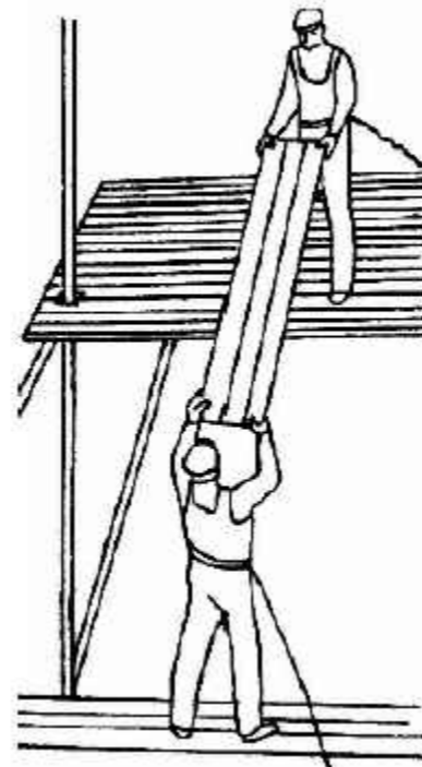
Розбирання щитового настилу
