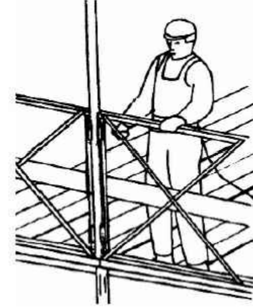
Зняття елементів огорожі на другому ярусі
