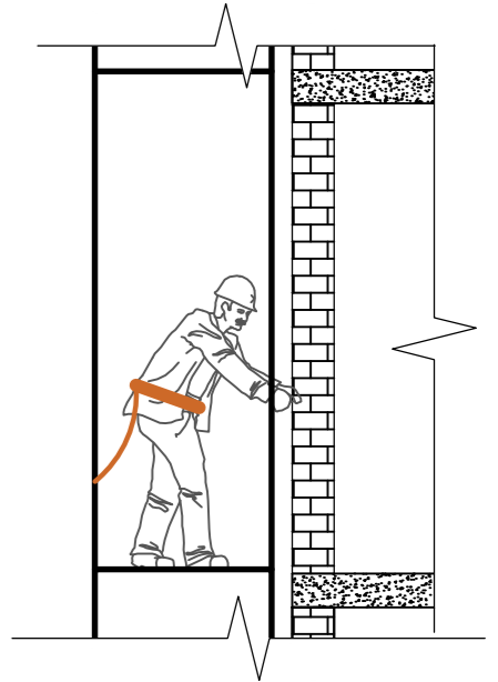
Кріплення страхуючого поясу до елементів риштувань
