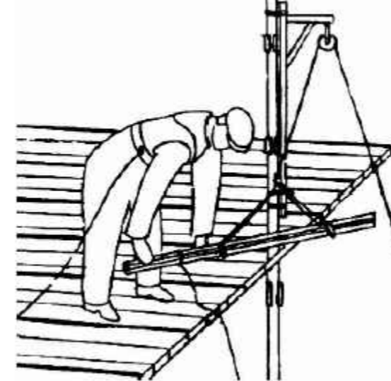
Спуск ригелів
