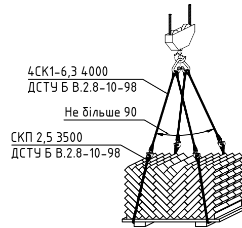
Схема стропування цегли на піддонах при розвантаженні транспортного засобу та подачі на площині складування матеріалів
