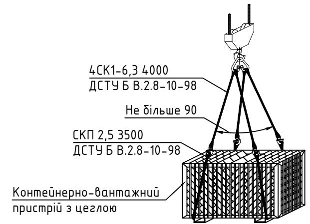
Схема стропування цегли на піддонах при розвантаженні транспортного засобу та подачі на площині складування матеріалів
