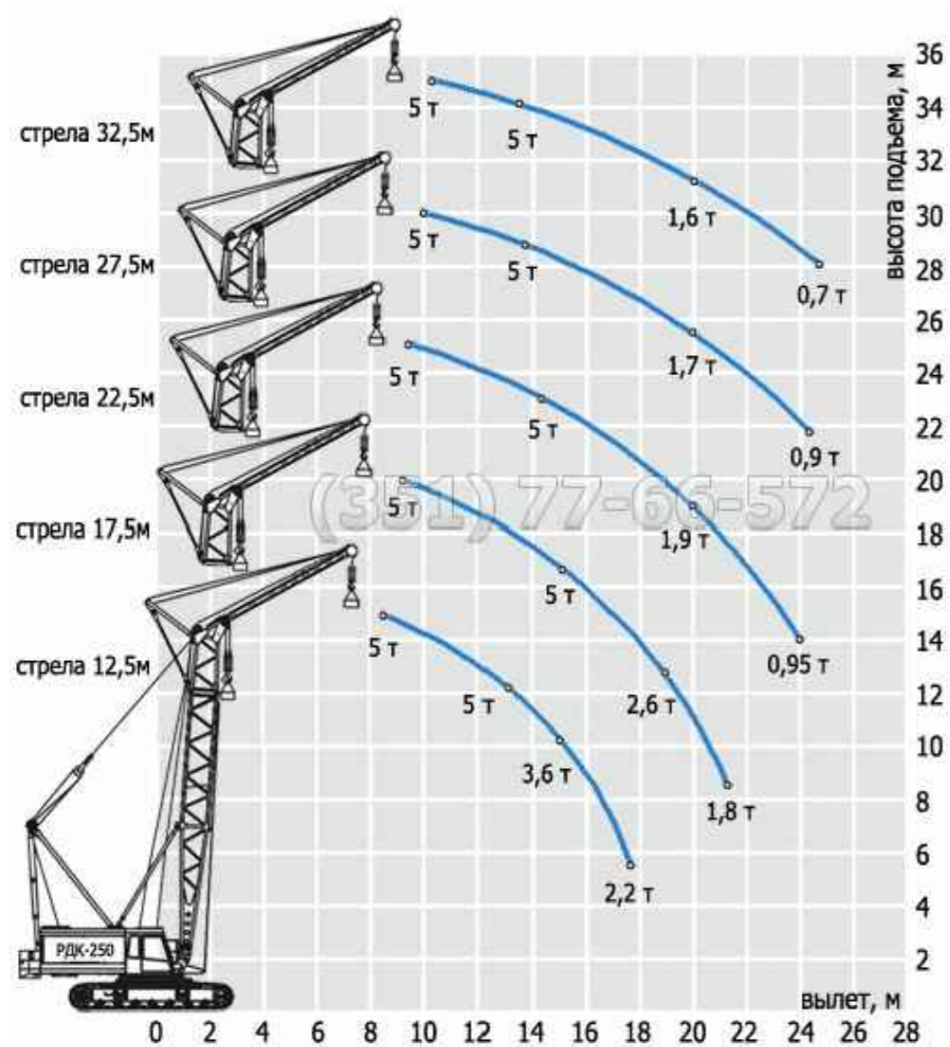
Вантажовисотні характеристики
